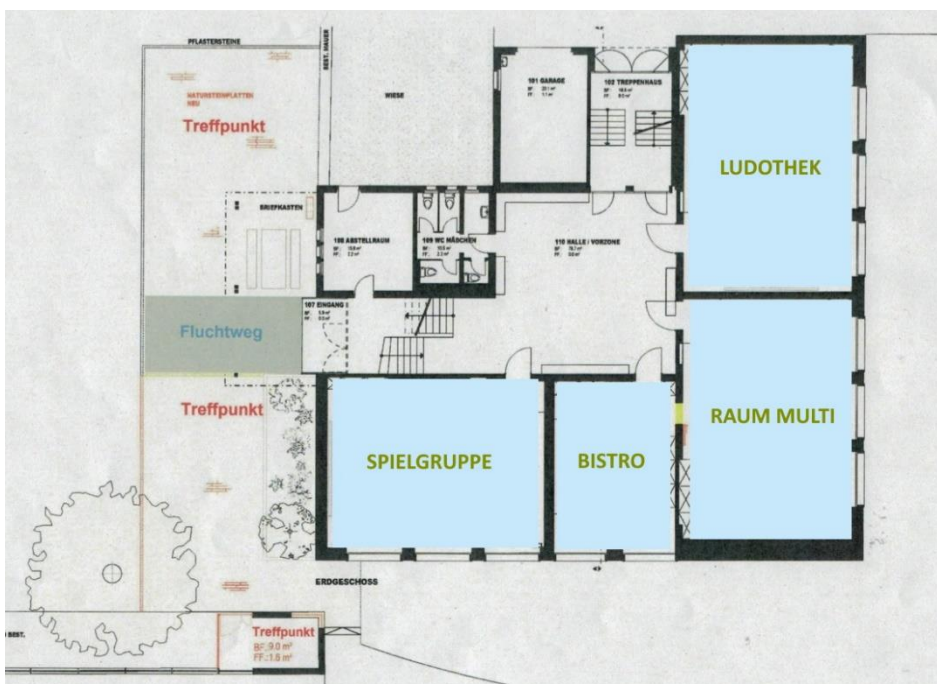
Grundriss Hochparterre, Altes Primarschulhaus Dorf, Meilen
